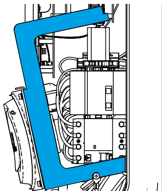
Image 5: Detachable subframe
